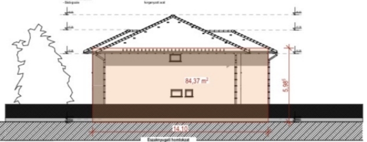
Északnyugati homlokzat
